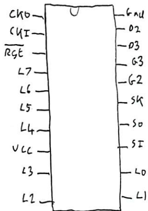
COP422 Microcontroller
